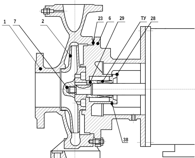
Насос с торцовым уплотнением
