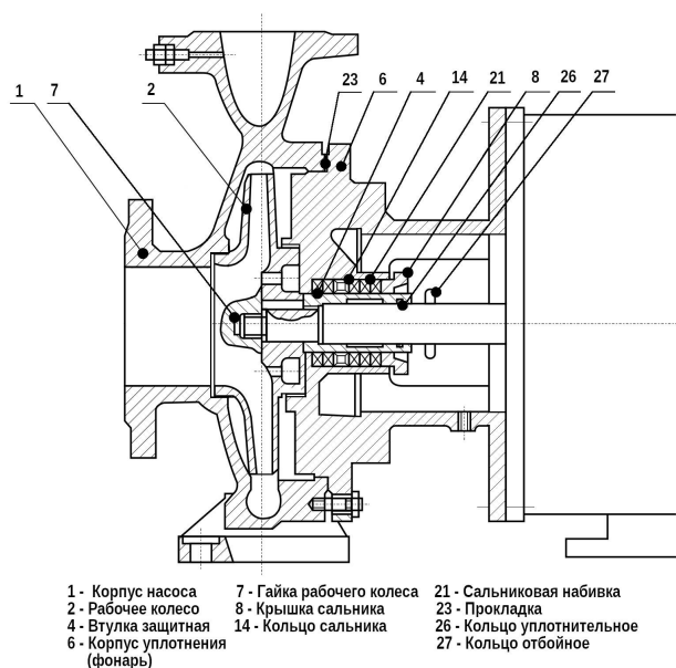
Насос с торцовым уплотнением
