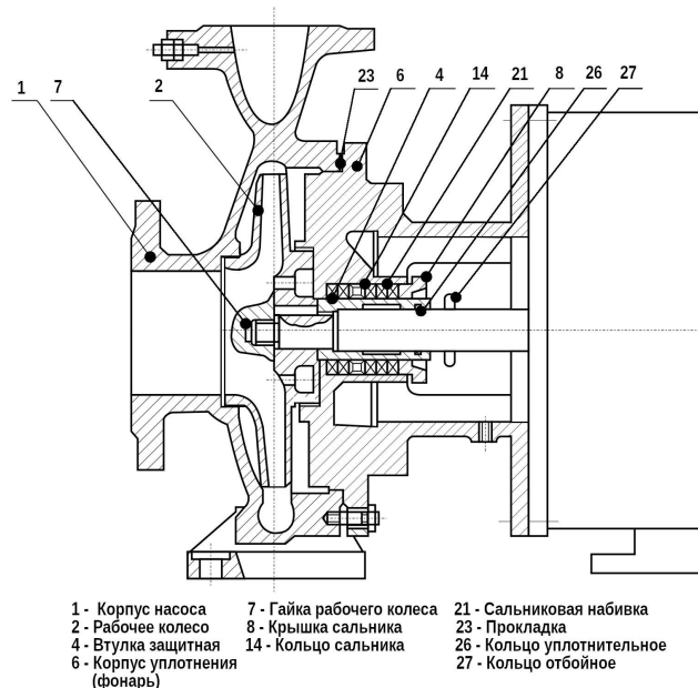
Насос с сальниковым уплотнением
