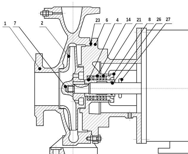
Насос с сальниковым уплотнением
