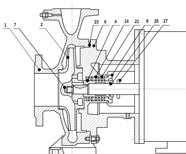
Насос с торцовым уплотнением
