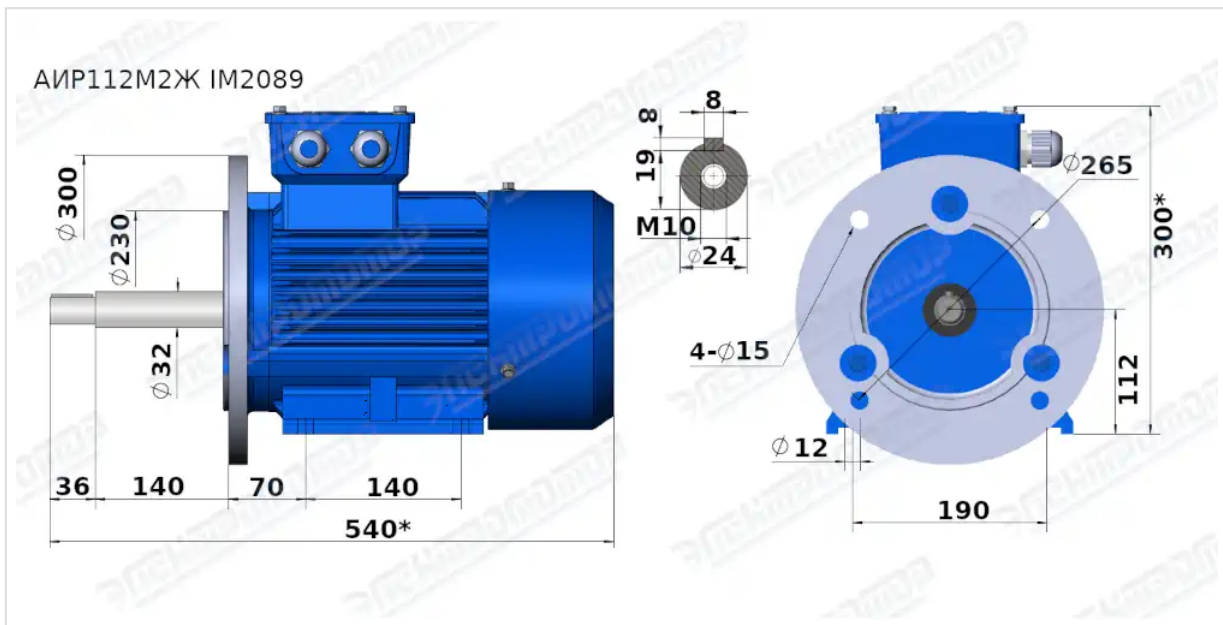
Чертеж АИР112М2 IM2089
